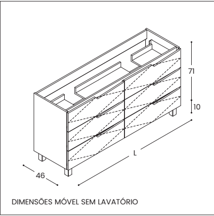
DIMENSÕES MÓVEL SEM LAVATÓRIO
